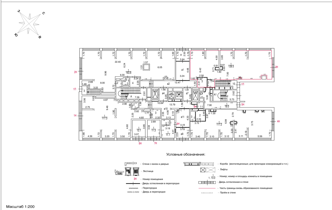
План здания, сооружения, план этажа, фрагмент плана здания, сооружения, этажа
